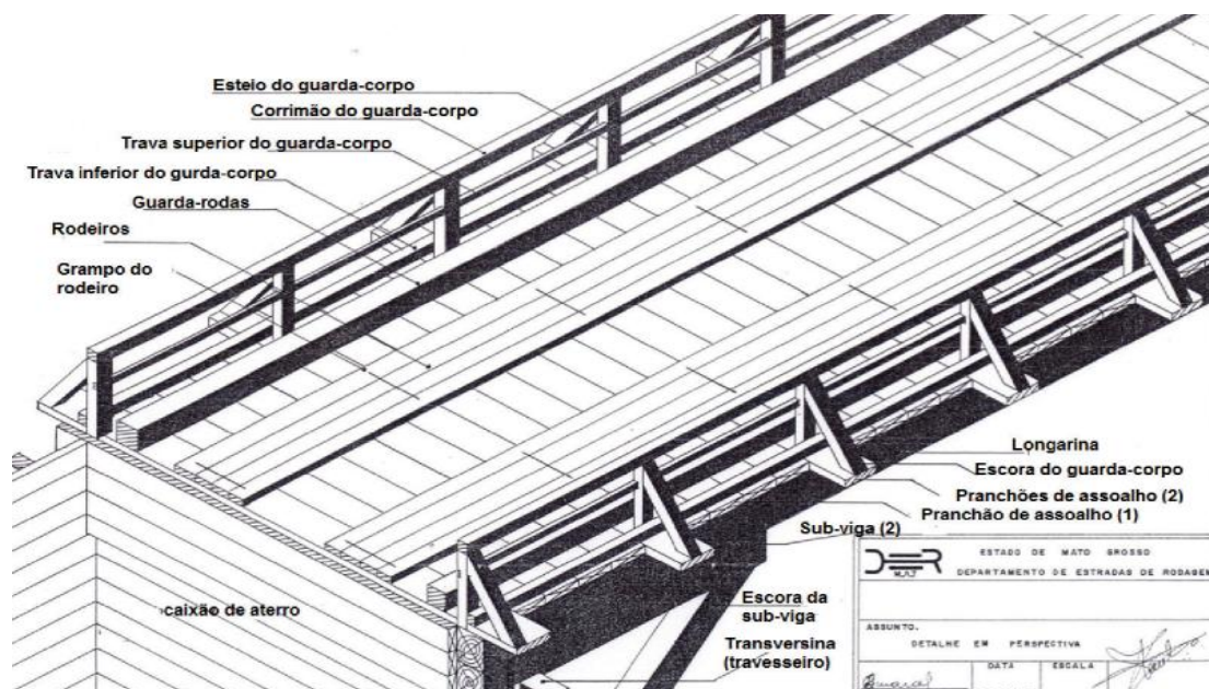
Figura 3: Imagem ilustrativa das partes estruturais de uma ponte de madeira; Fonte: DERMAT (1979).
